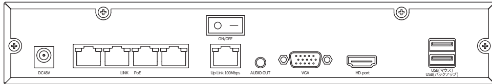
NVR(ネットワークビデオレコーダー) 4CH裏面
