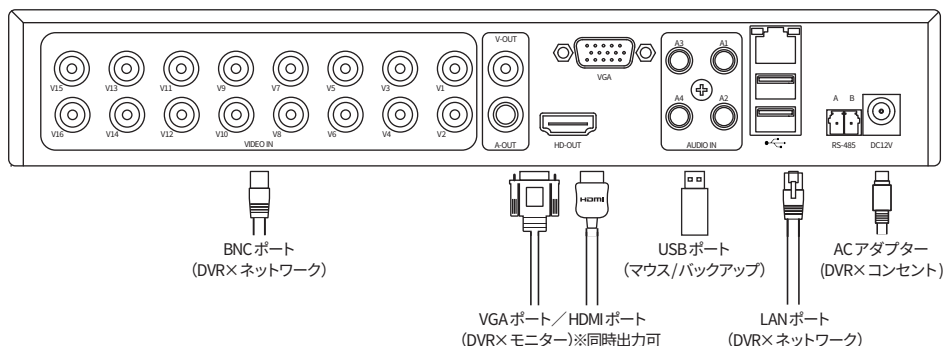
DVR(デジタルビデオレコーダー) 16CH 裏面※別売
